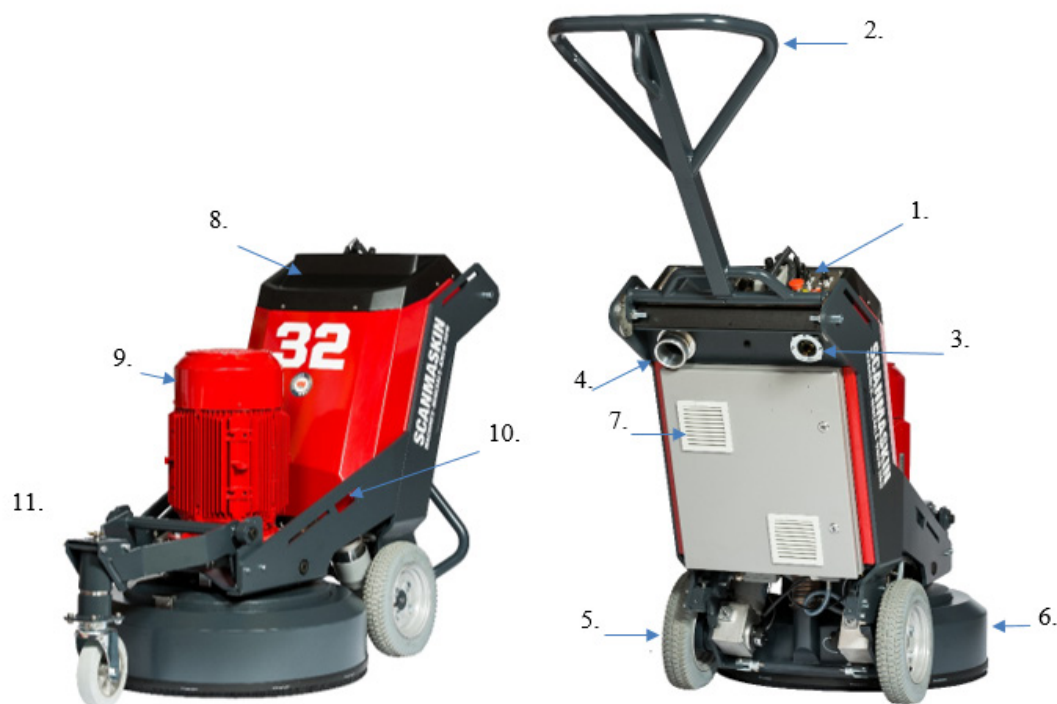
Figur 13 Översikt över SCANMASKIN 32 WS
