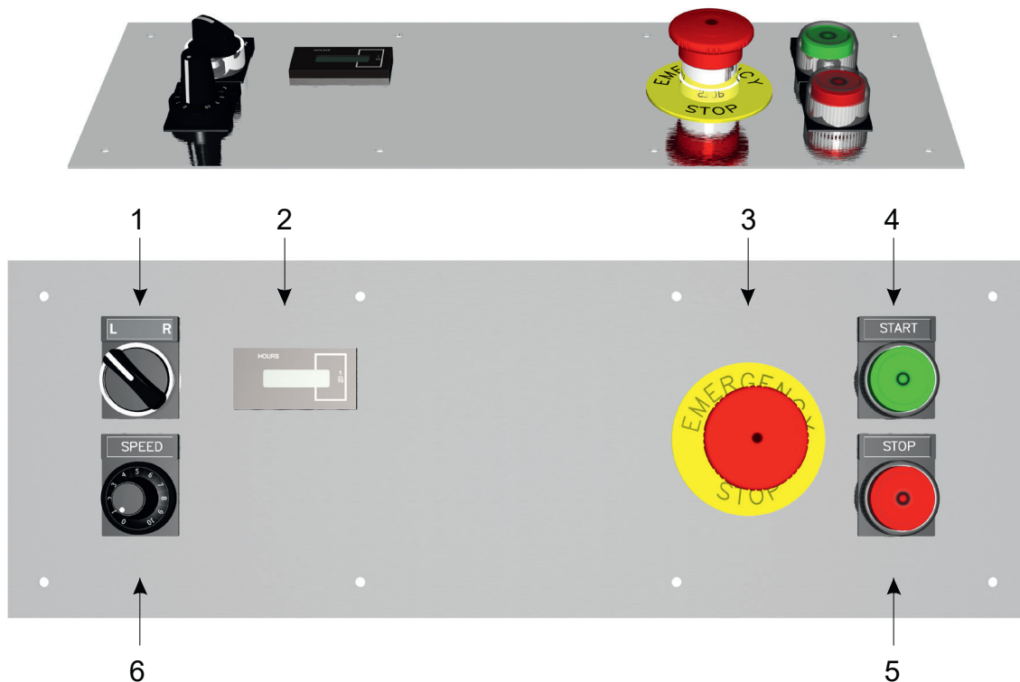
Figur 4.2 SC-650 kontrollpanel
