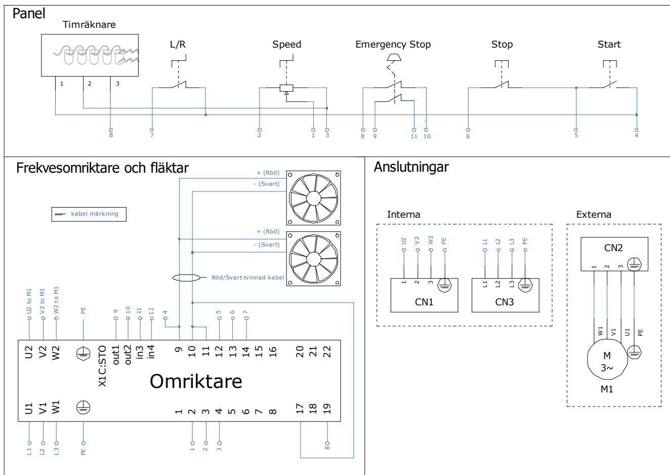
Figur 61 Elschema SC-650
