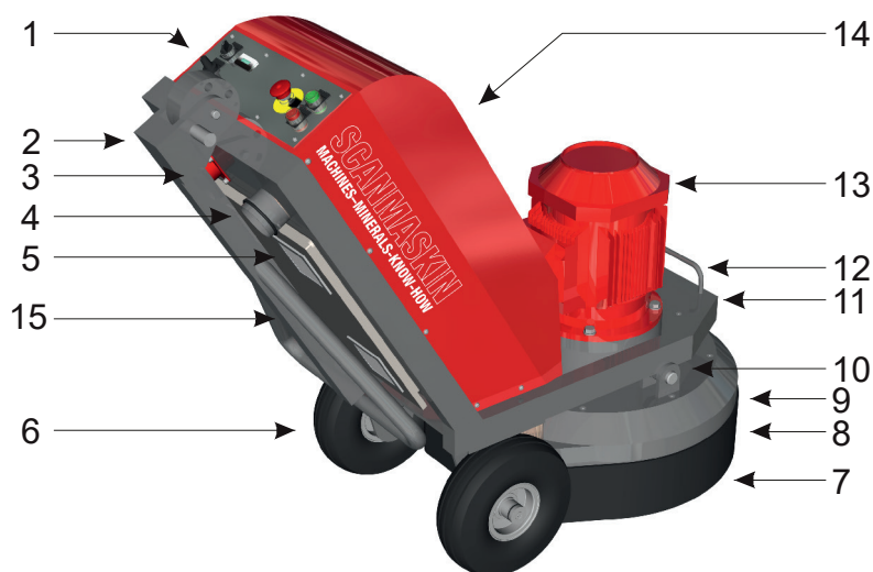
Figur 1.3 SC-650 översikt
